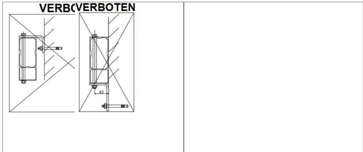
Zeichn. 33B – Universalwandhalter – Verbotene Montagearten
