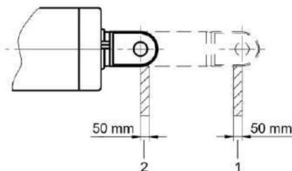
Zeichn. 30 Zulässige Hubreduktion
